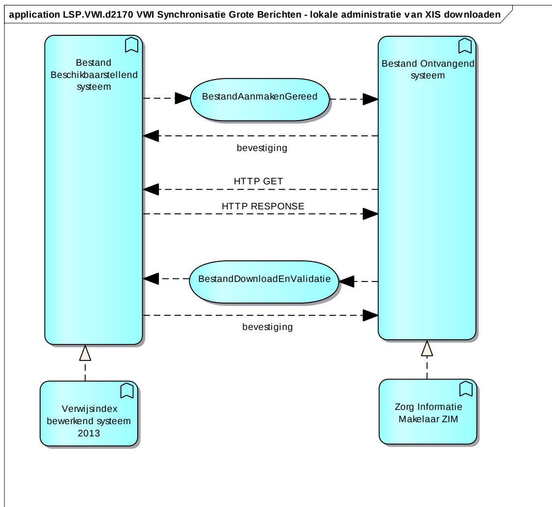
Diagram LSP.VWI.d2170 – Afhandelen van interface Synchroniseren indexgegevens – lokale administratie van XIS downloaden
