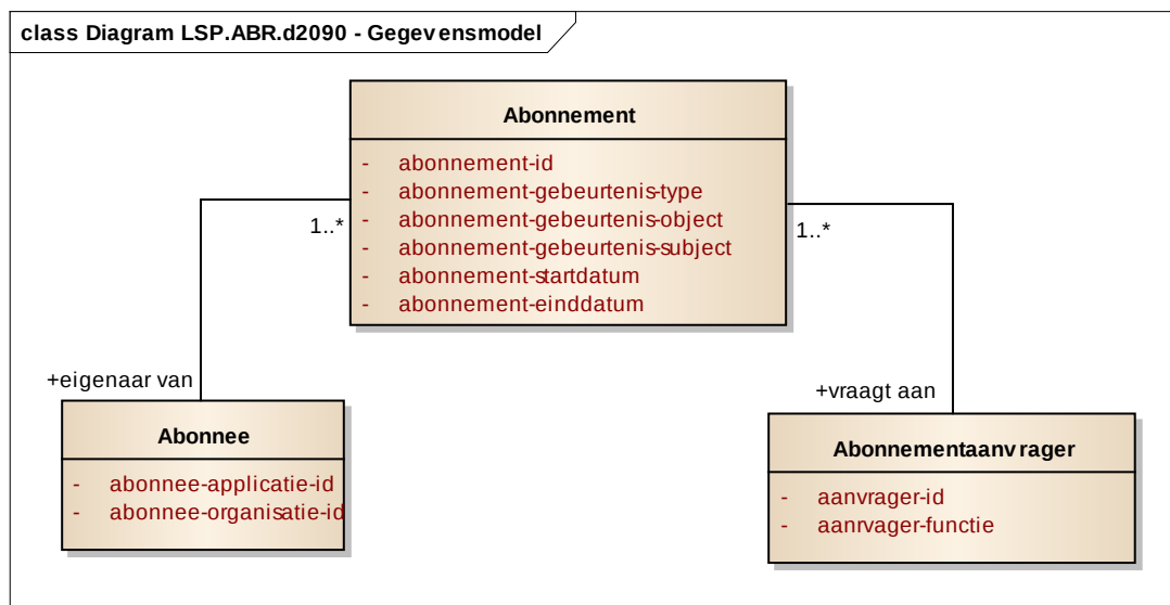
Diagram LSP.ABR.d2090 – Gegevensmodel
