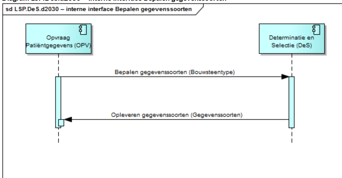
Diagram LSP.DeS.d2030 – interne interface Bepalen gegevenssoorten
